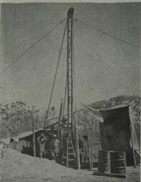
Camino de Achaguas, el Gobierno Nacional hace la perforación de estos pozos para obtener agua potable.
