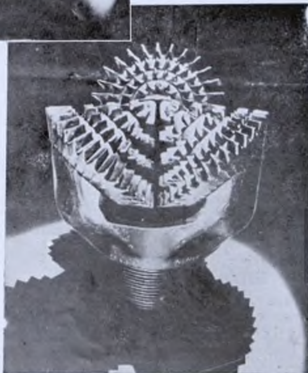
Mecha de RACHET, de tres piñones, para roca dura.
